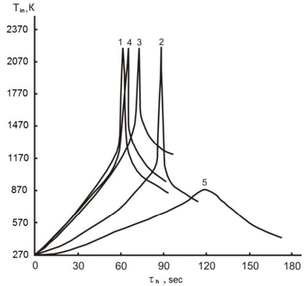
1 – 0,86 Ti + Si, T_{in} = 1270 K; 2 – 0,86 Ti + Si + 0.005 S, T_{in} = 1070 K;
